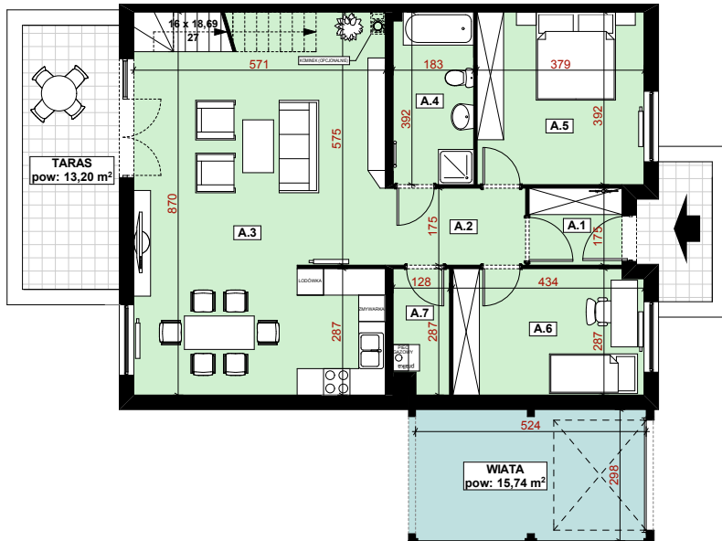
RZUT PARTERU
