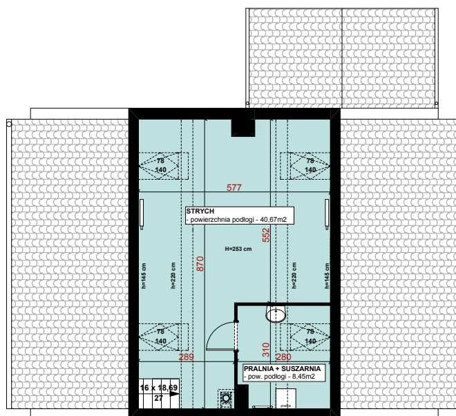
RZUT PODDASZA
