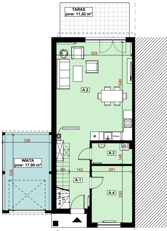
RZUT PARTERU
