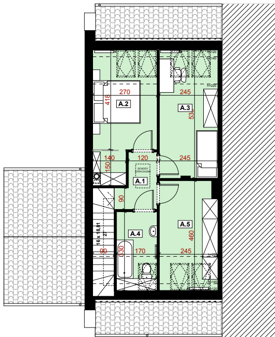
RZUT PODDASZA
